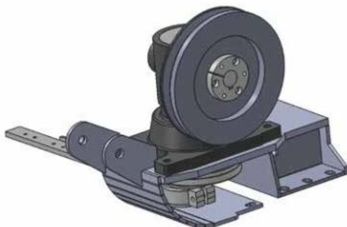
CONJUNTO ADAPTACIÓN CASE CON PLATAFORMA 3020 IZQUIERDA Y DERECHA
