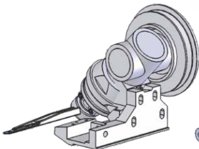
CONJUNTO ADAPTACIÓN JOHN DEERE 9650 DERECHA - PARA CMU 2000
