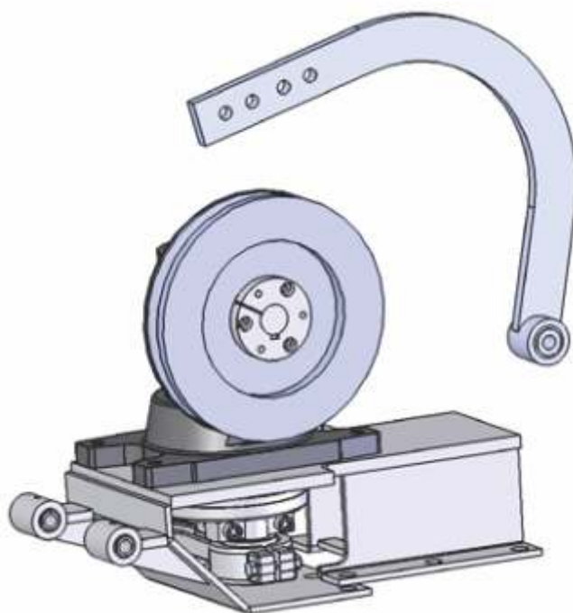
CONJUNTO ADAPTACIÓN CASE 2388
